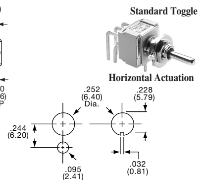
SPDT
